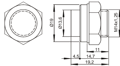
Dimensiones del rácor engrapado M14x1'25
